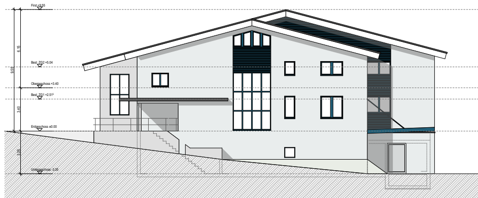
Ostfassade
